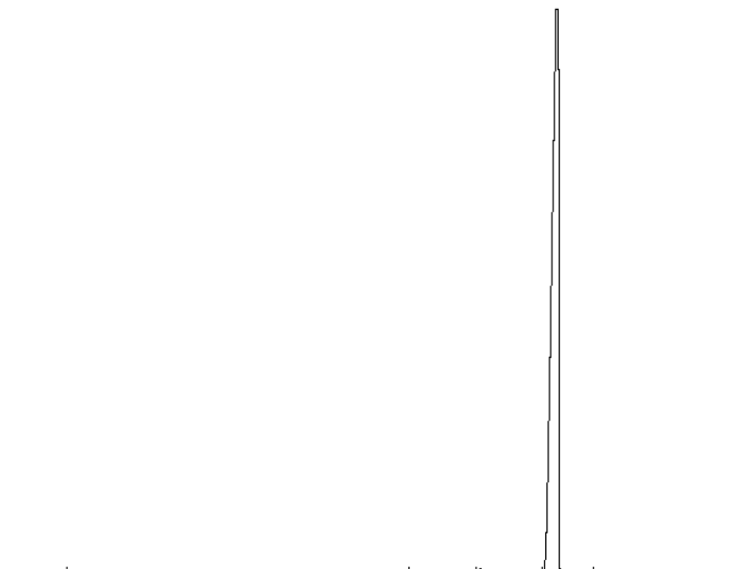
图 B.1 食品添加剂丁酰乳酸丁酯典型气相色谱图
